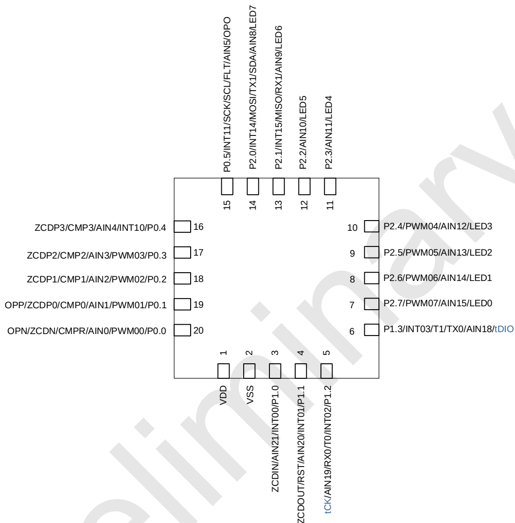
SC92R349 管脚配置图 适用于 QFN20 封装
