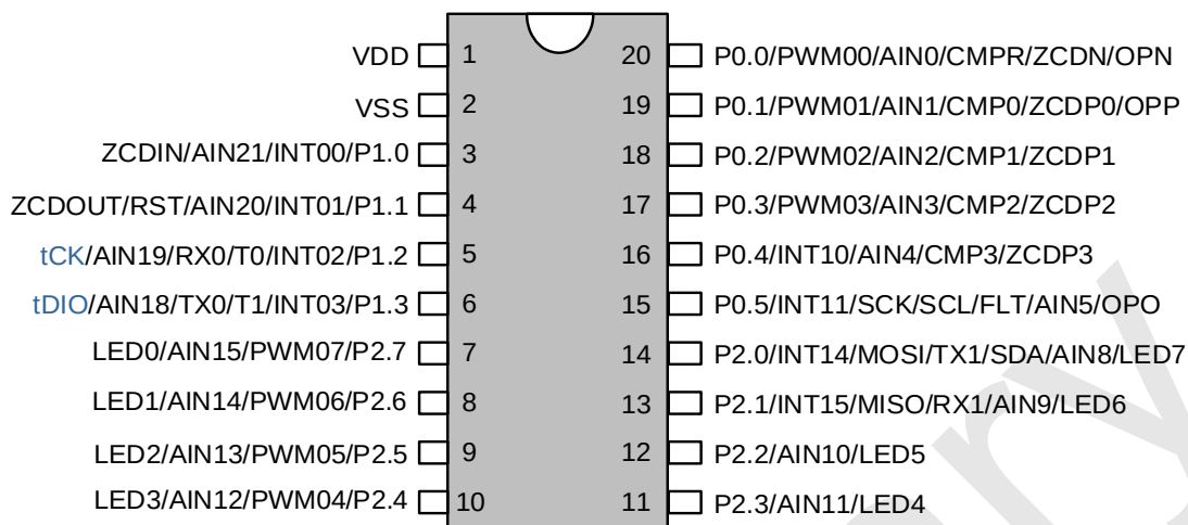
SC92R349 管脚配置图 适用于 SOP20/TSSOP20 封装
