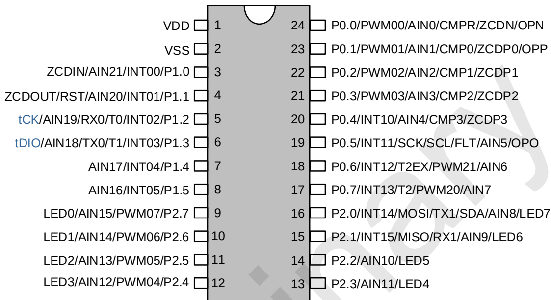
SC92R349 管脚配置图 适用于 SSOP24 封装
