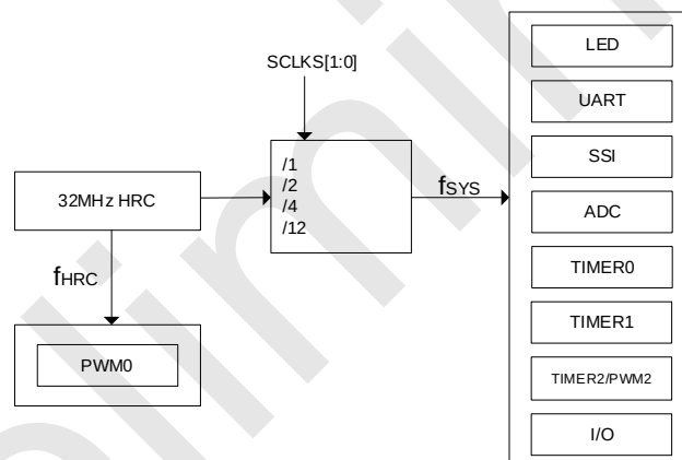
SC92R349 内部时钟关系
