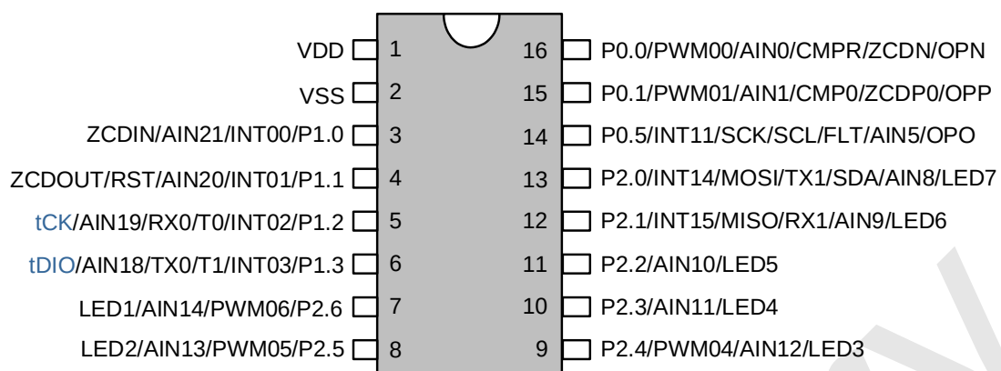
SC92R349 管脚配置图 适用于 SOP16 封装
