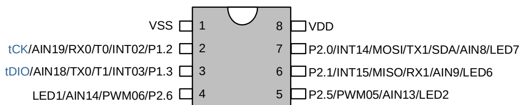
SC92R349 管脚配置图 适用于 SOP8 封装
