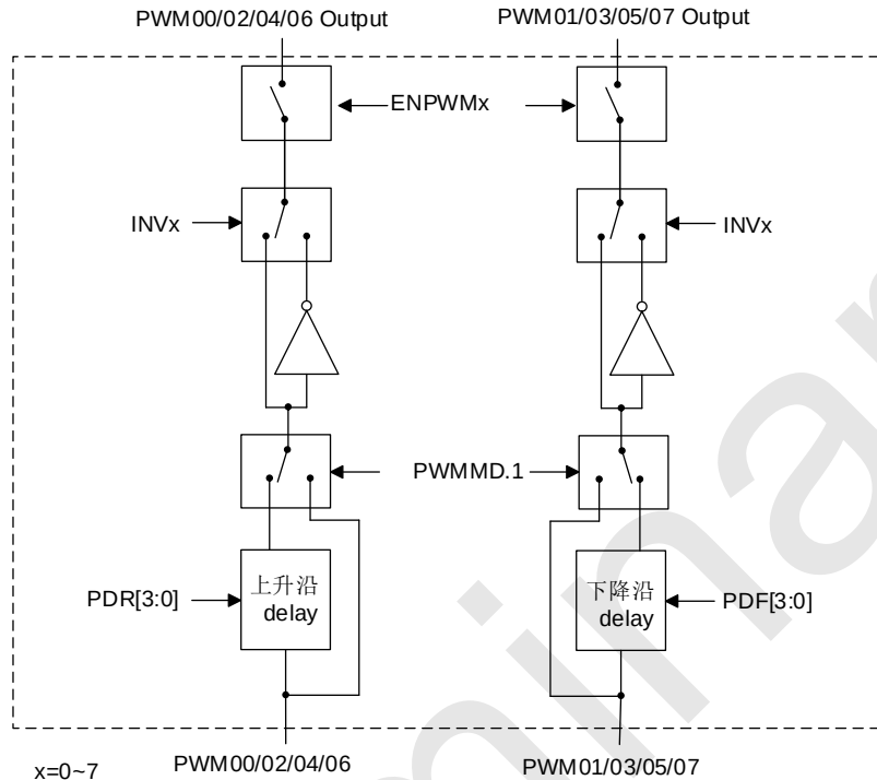
SC92R349 PWM 互补模式框图
